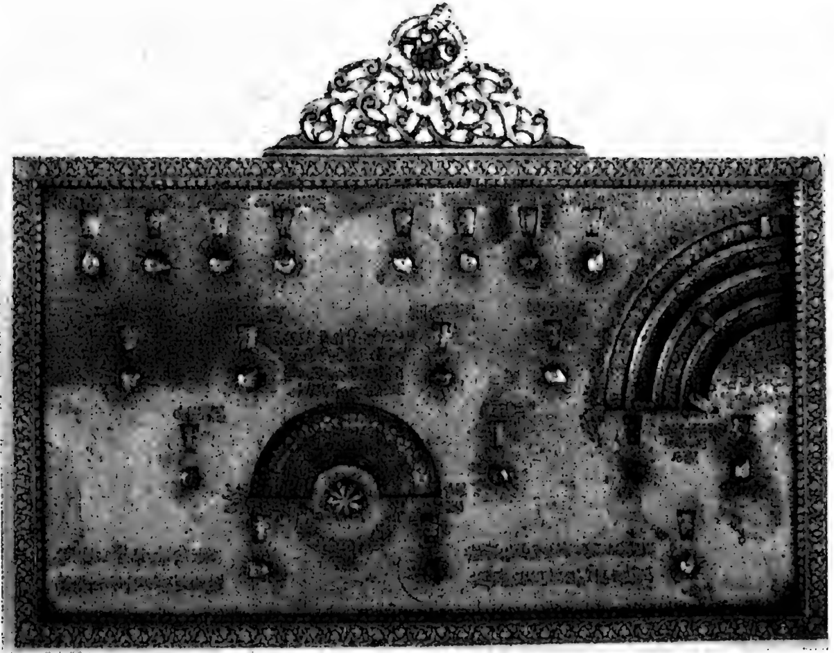
الصرورة ١٨-٨ آلة هندسية من سوريا أو من بلاد ما بين النهرين مصنوعة من النحاس الأصفر والأحمر، مطعمة بالفضة والذهب، بتوقيع (محمد بن ختلخ الموصلي) بتاريخ ٦٩٣ هـ / ١٢٤١ م. [بترخيص من المتحف البريطاني - لندن].
